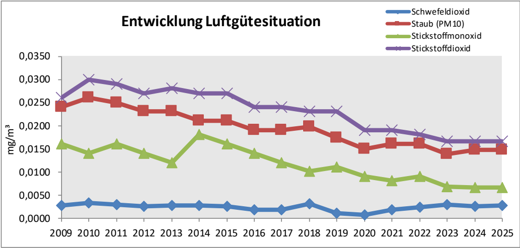
Abb. 23: Entwicklung Luftgütesituation
