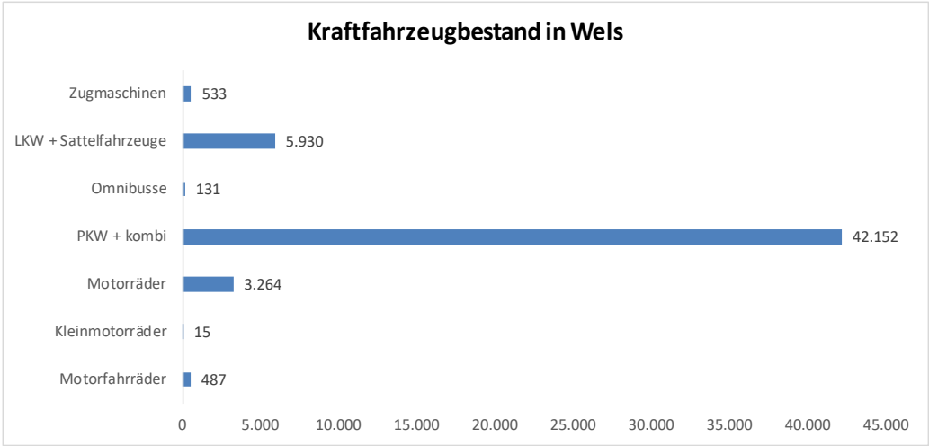
Abb. 40: Kraftfahrzeugsbestand
