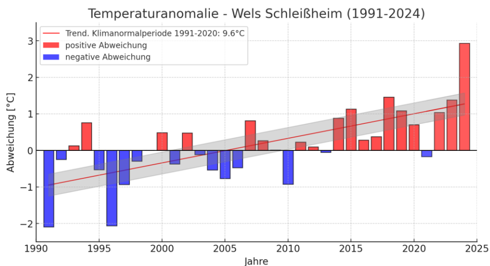
Abbildung 6: Temperaturanomalie der Klimanormalperiode 1991-2020, Abweichungen bis zum Jahr 2024, eigene Darstellung. Datenquelle: GeoSphereAustria
