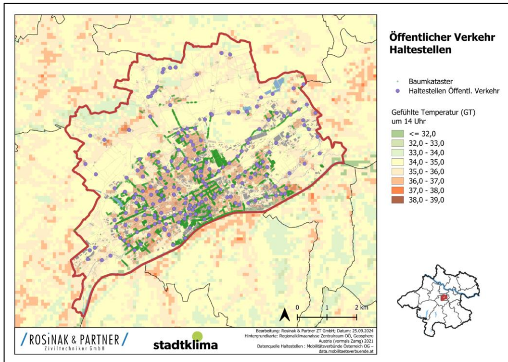
Abbildung 15: Gefühlte Temperatur um 14 Uhr, überlagert mit dem Baumkataster und den Haltestellen des öffentlichen Verkehrs. Datenquelle: Regionalklimaanalyse Zentralraum OÖ
