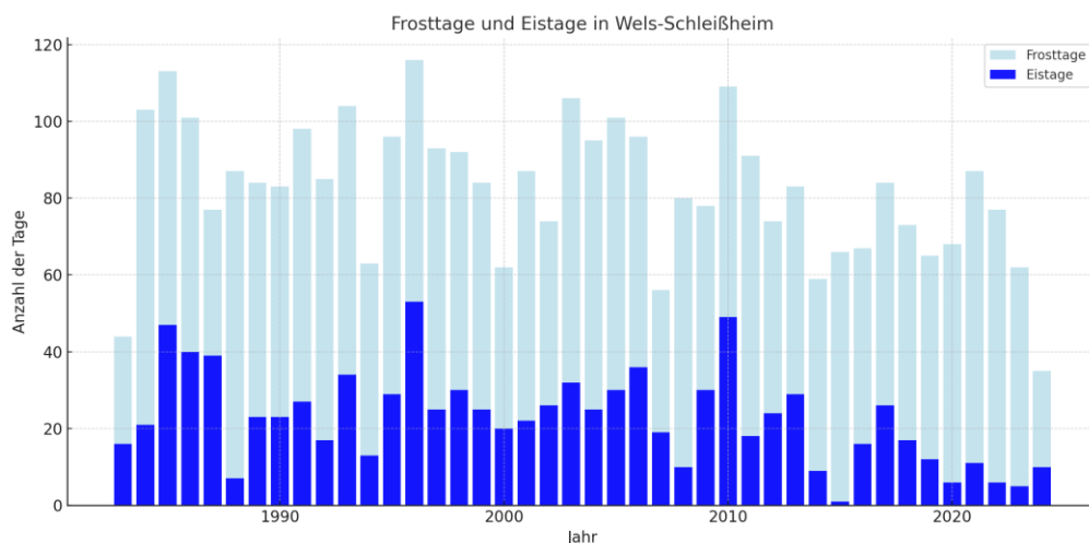
Abbildung 9: Anzahl der jährlich auftretenden Frost- und Eistage seit 1983, eigene Darstellung. Datenquelle: GeoSphere Austria
