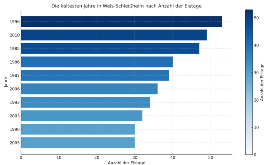
Abbildung 10: Rangliste der 10 häufigsten Eistage seit 1983, eigene Darstellung. Datenquelle: GeoSphere Austria
