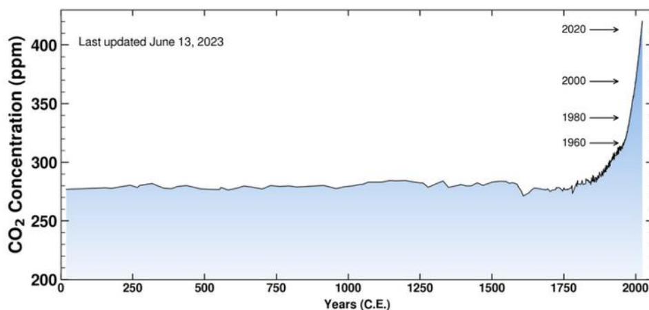
Abbildung 1: Entwicklung der CO 2 Konzentration auf der Erde (Quelle: Scripps Institution of Oceanography, UC San Diego)
