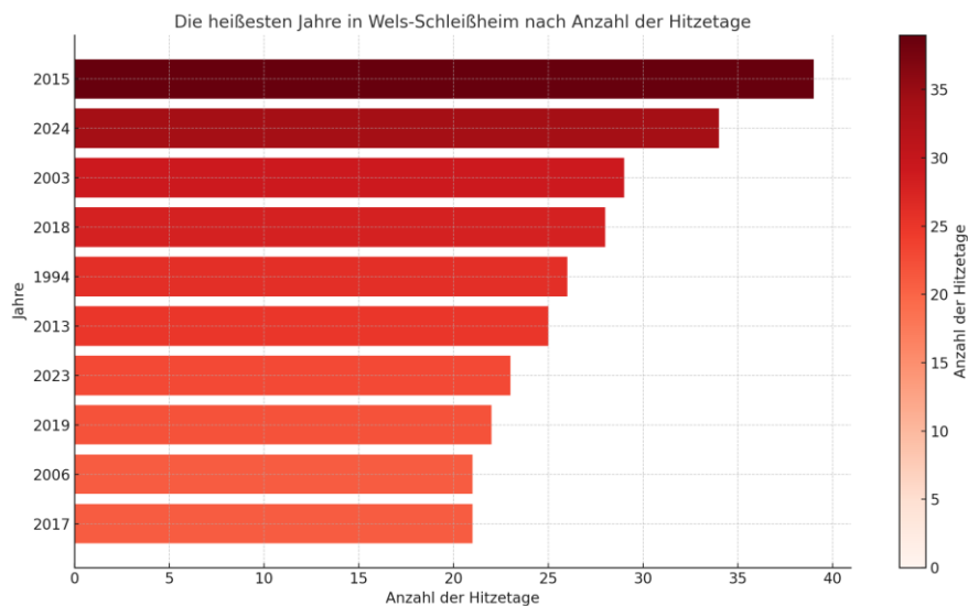
Abbildung 8: Rangliste der 10 häufigsten Hitzetage seit 1983, eigene Darstellung. Datenquelle: GeoSphere Austria
