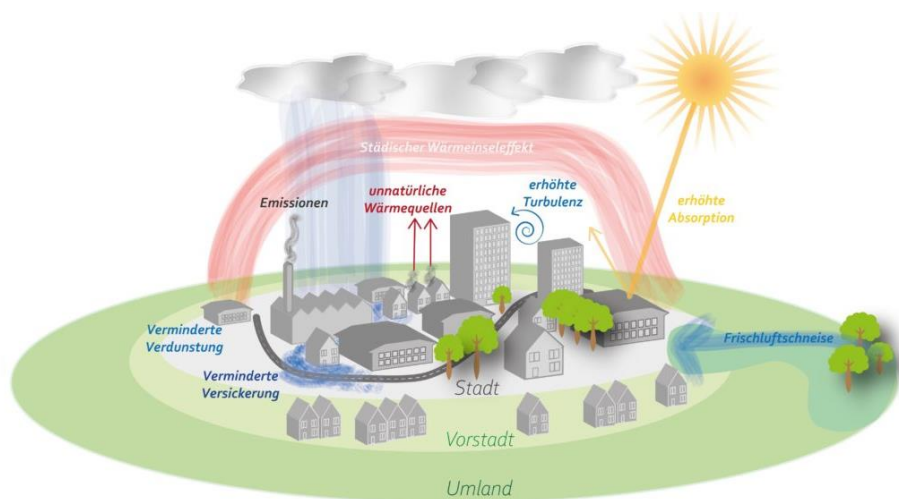
Abbildung 4: Schematische Darstellung des Effekts der städtischen Wärmeinsel (Quelle: Stadt Herten 2020)
