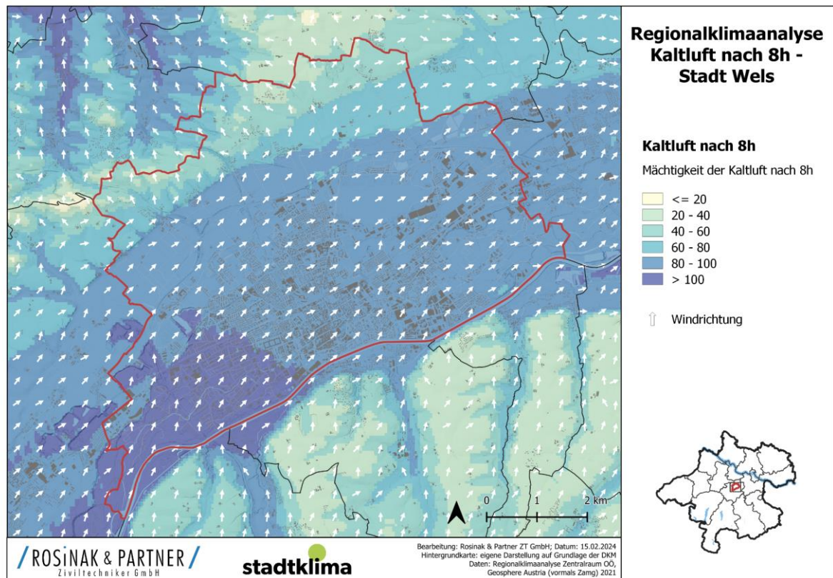
Abbildung 12: Darstellung der Kaltluftparameter acht Stunden nach Sonnenuntergang. Datenquelle: Regionalklimaanalyse Zentralraum OÖ
