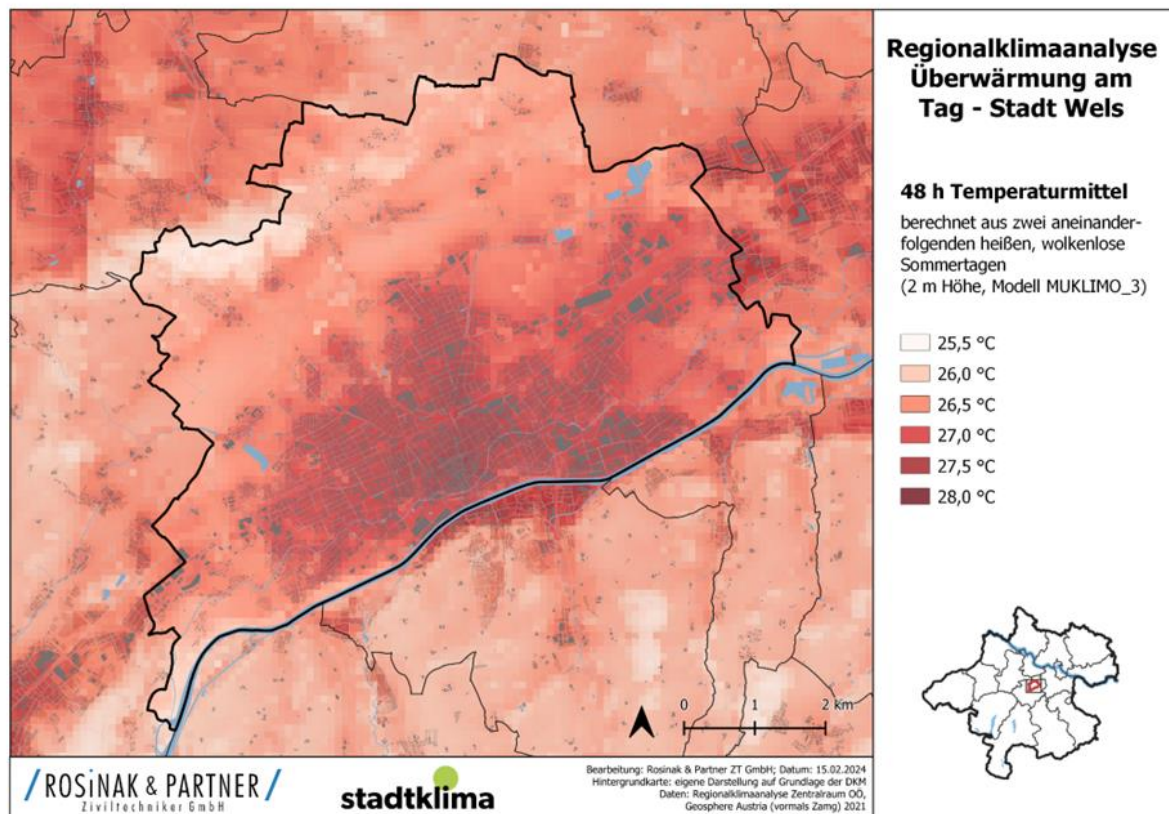
Abbildung 13: Darstellung der Überwärmung für die Stadt Wels. Datenquelle: Regionalklimaanalyse Zentralraum OÖ
