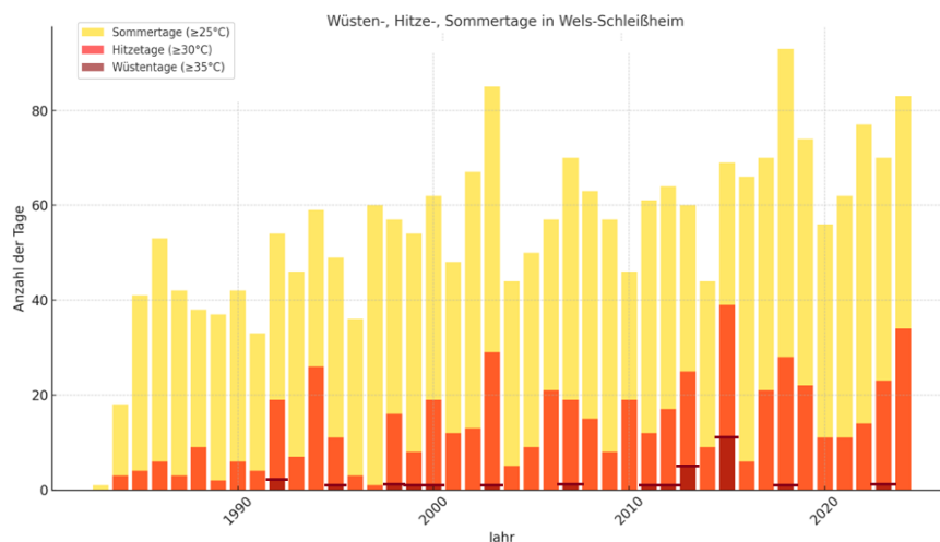
Abbildung 7: Anzahl der jährlich auftretenden Wüsten-, Hitze- und Sommertage seit 1983, eigene Darstellung. Datenquelle: GeoSphere Austria
