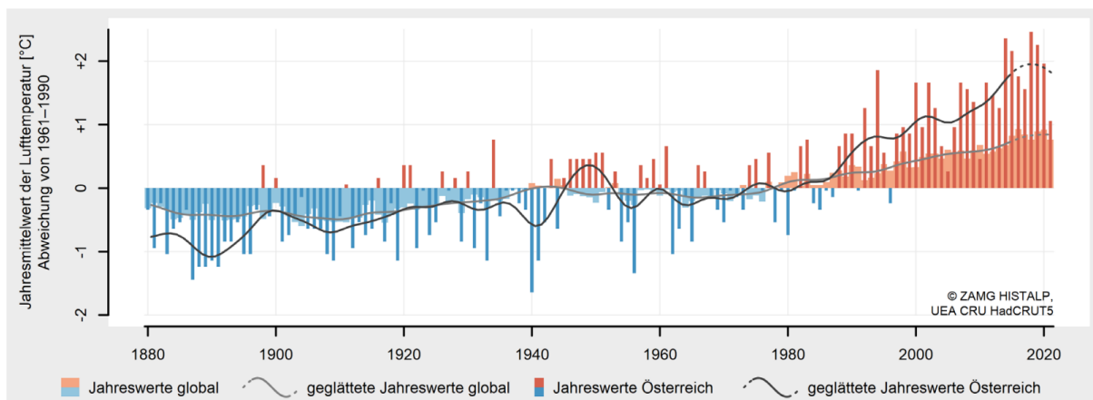
Abbildung 5: Langfristige Entwicklung der Jahreswerte der Lufttemperatur global und in Österreich von 1880 bis 2021. Dargestellt sind Abweichungen von den jeweiligen Mittelwerten des Bezugszeitraumes 1961–1990. (Quelle: Stangl et al. 2022)
