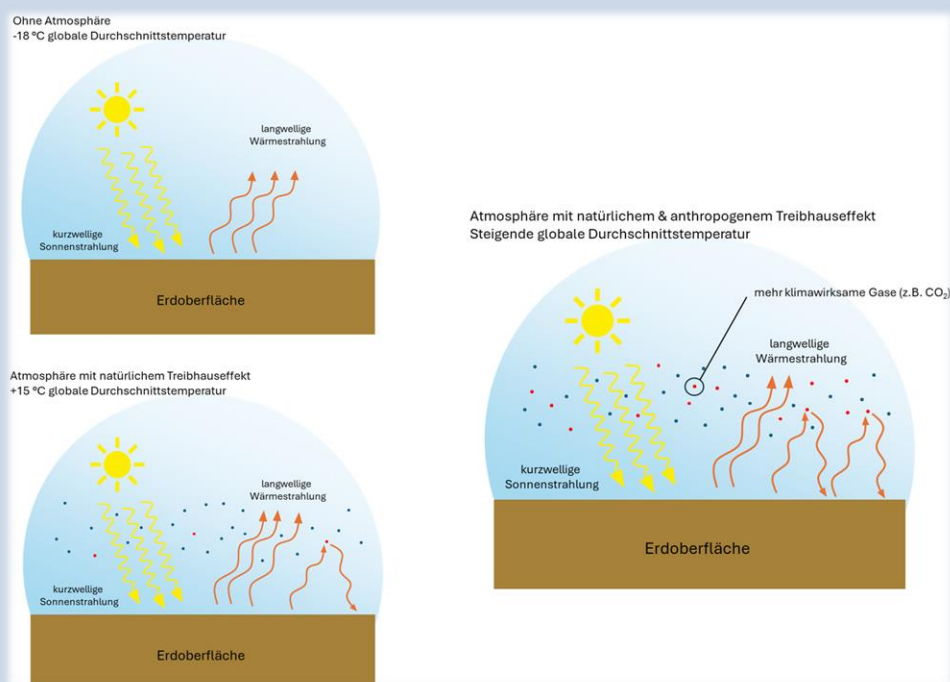
Abbildung 2: Vereinfachte Darstellung des Treibhausgaseffekts, eigene Darstellung
